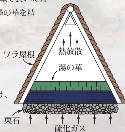
湯の華小屋構造図
