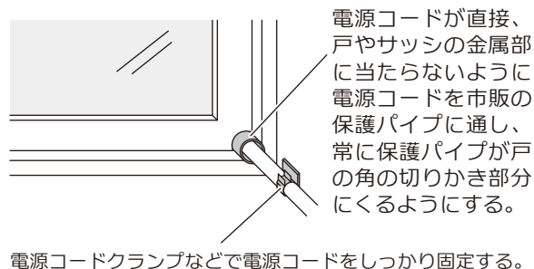
例 4. 窓に電線通し板を設け、屋外のコンセントを利用する場合
