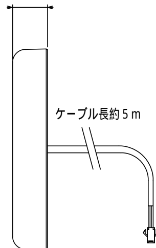
【側面図】
